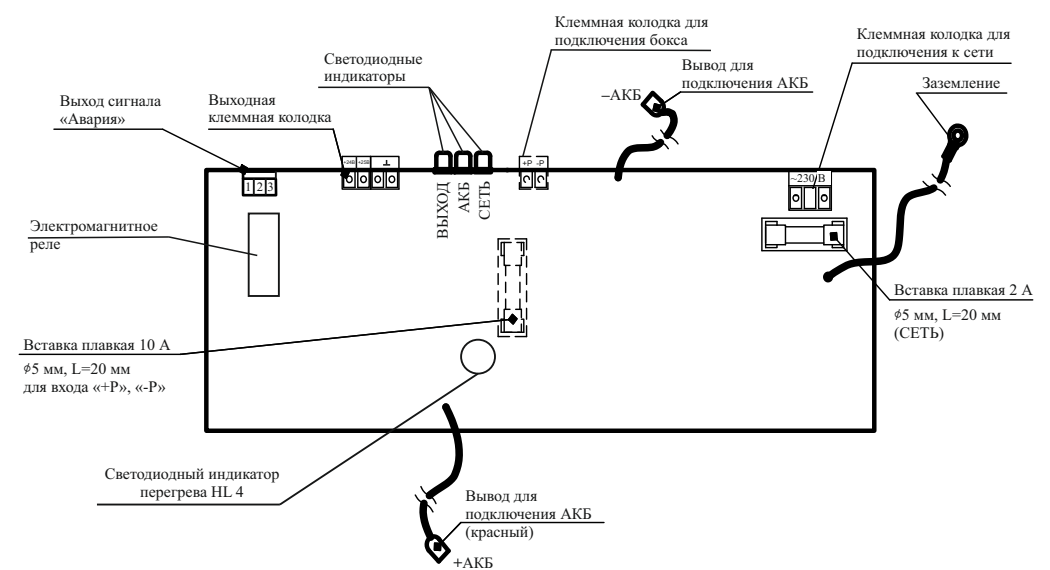
Рисунок 1 – Плата источника
