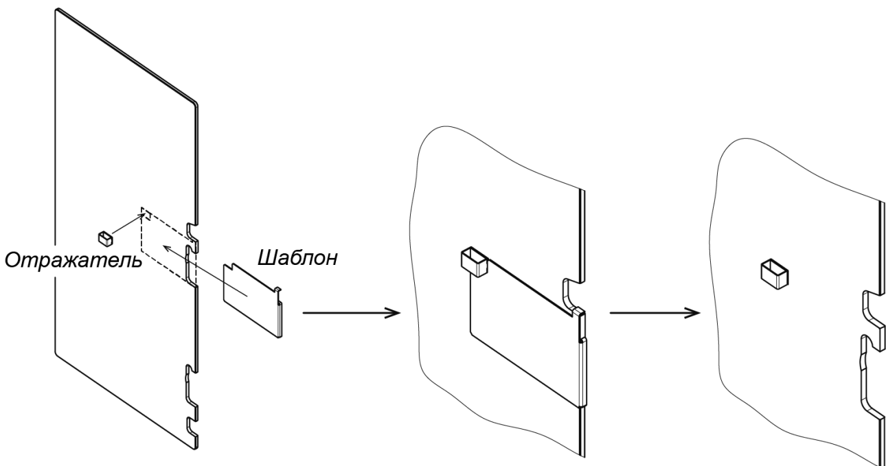
Рисунок 28. Установка отражателя
