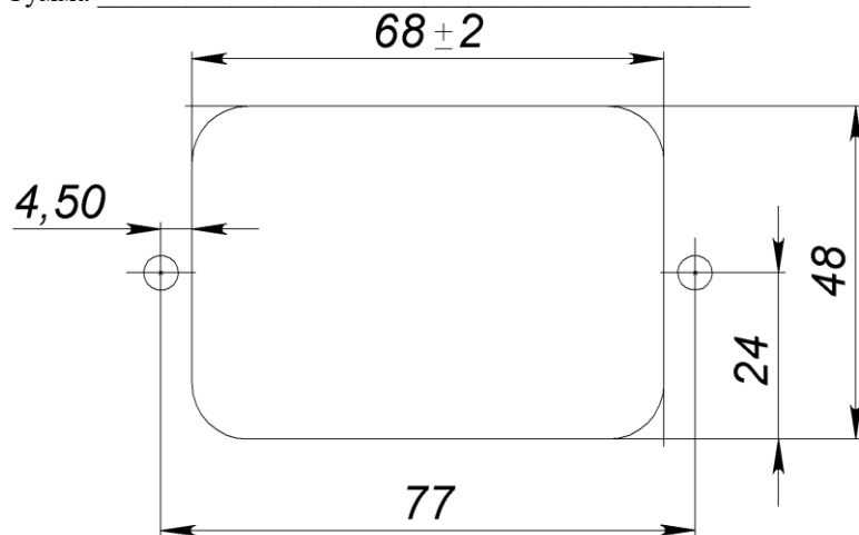
Рис2. Разметка под установку видеокамеры EVM1-IP2-IRM
