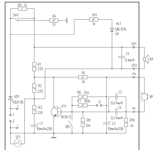
Схема электрическая принципиальная ТАП ЦИФРАЛ КМ-3
