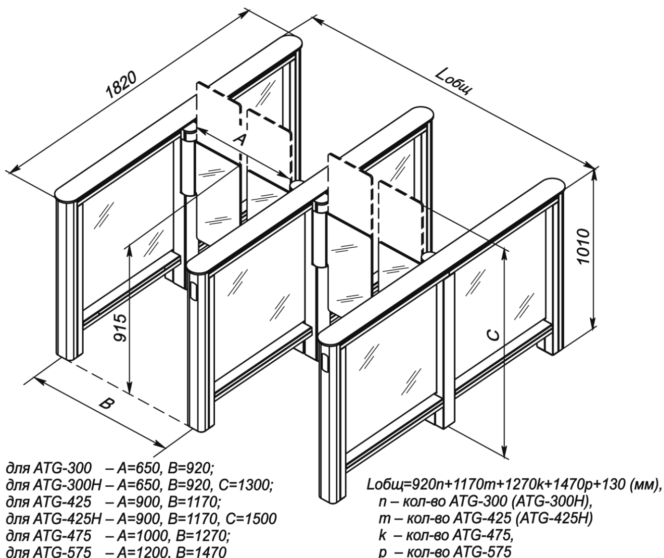
Рисунок 7. Габаритные размеры турникета при организации нескольких зон прохода
