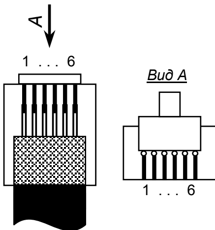
Рис. 2. Разъем
