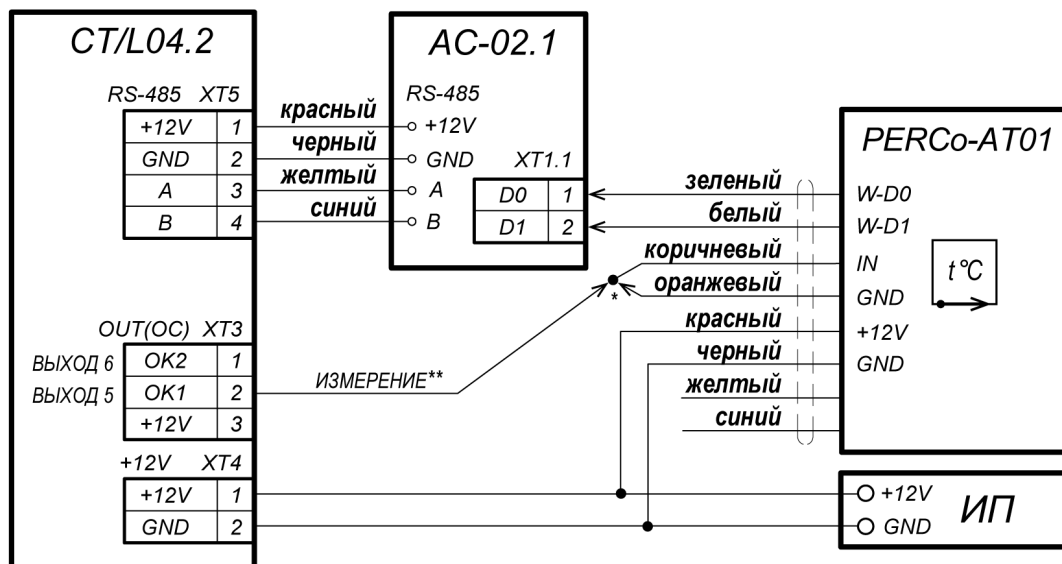
Рисунок 24. Схема подключения к контроллеру CT/L04.2 пирометра PERCo-AT01 с конфигурацией «ВВУ с тактированием»
