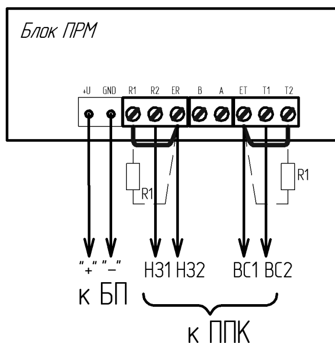
Рисунок 2.6 – Подключение ПРМ с отдельным выводом цепей реле (НЗ) и вскрытия (ВС)
