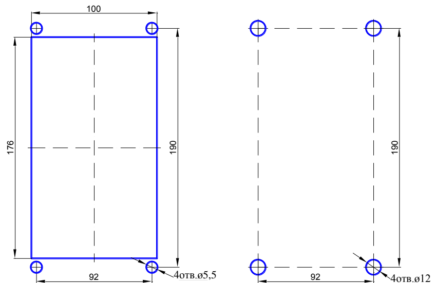
Рис1. Разметка под крепление DP300-TD22 а) снаружи; б) изнутри.
