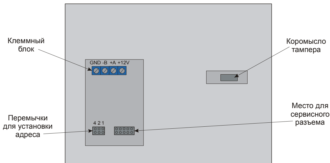
Рисунок 2. Вид клавиатуры АКД-01 сзади.
