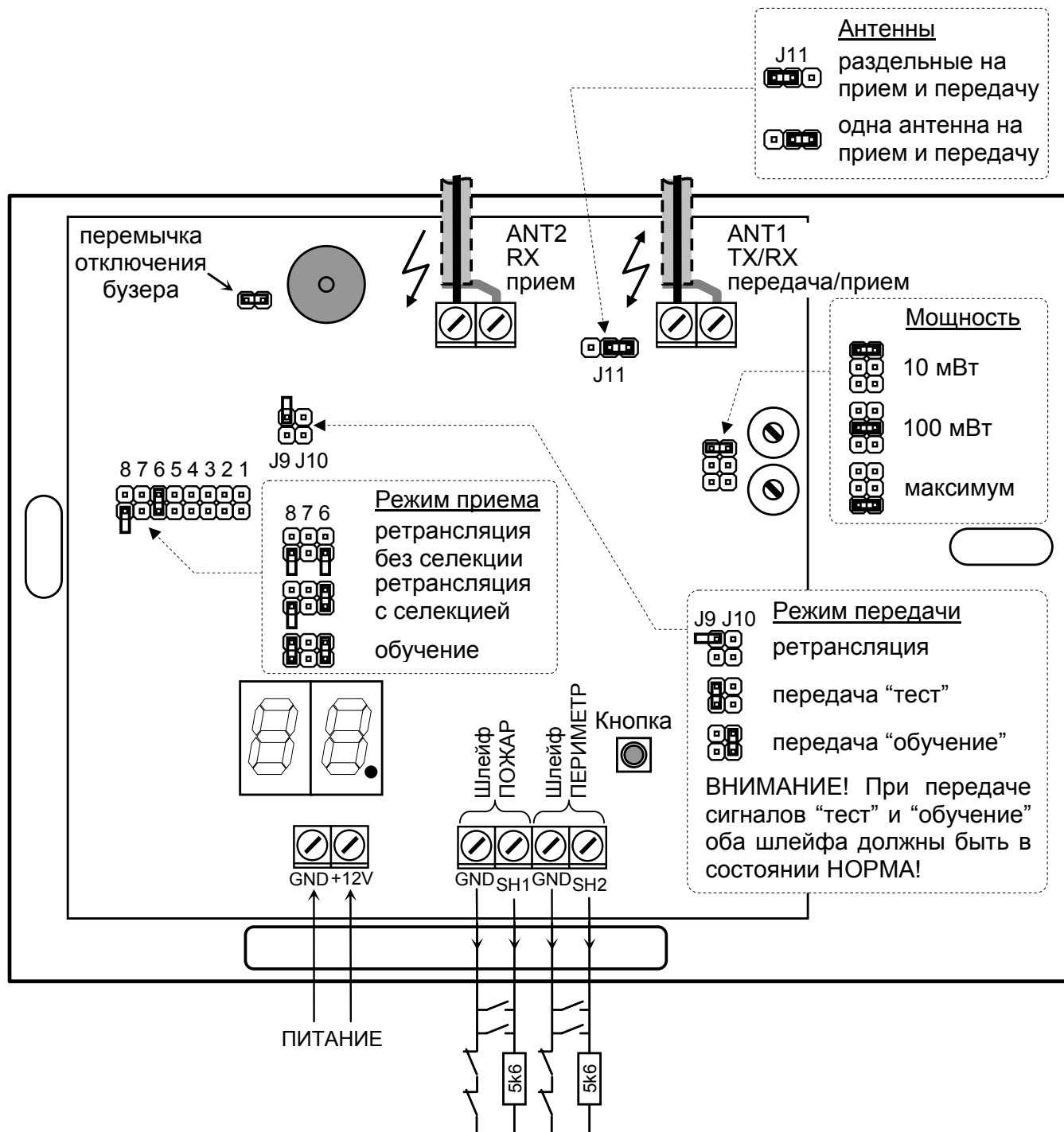
Рис. 3. Монтажная схема ретранслятора
