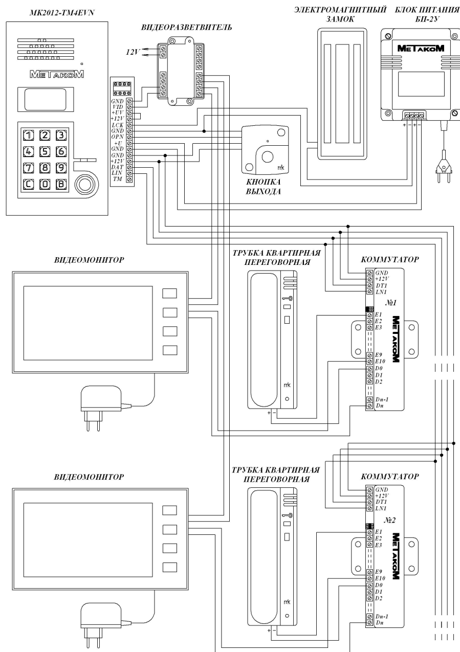
Рис. 2 Пример монтажа блока вызова МК2012-ТМ4ЕVН
