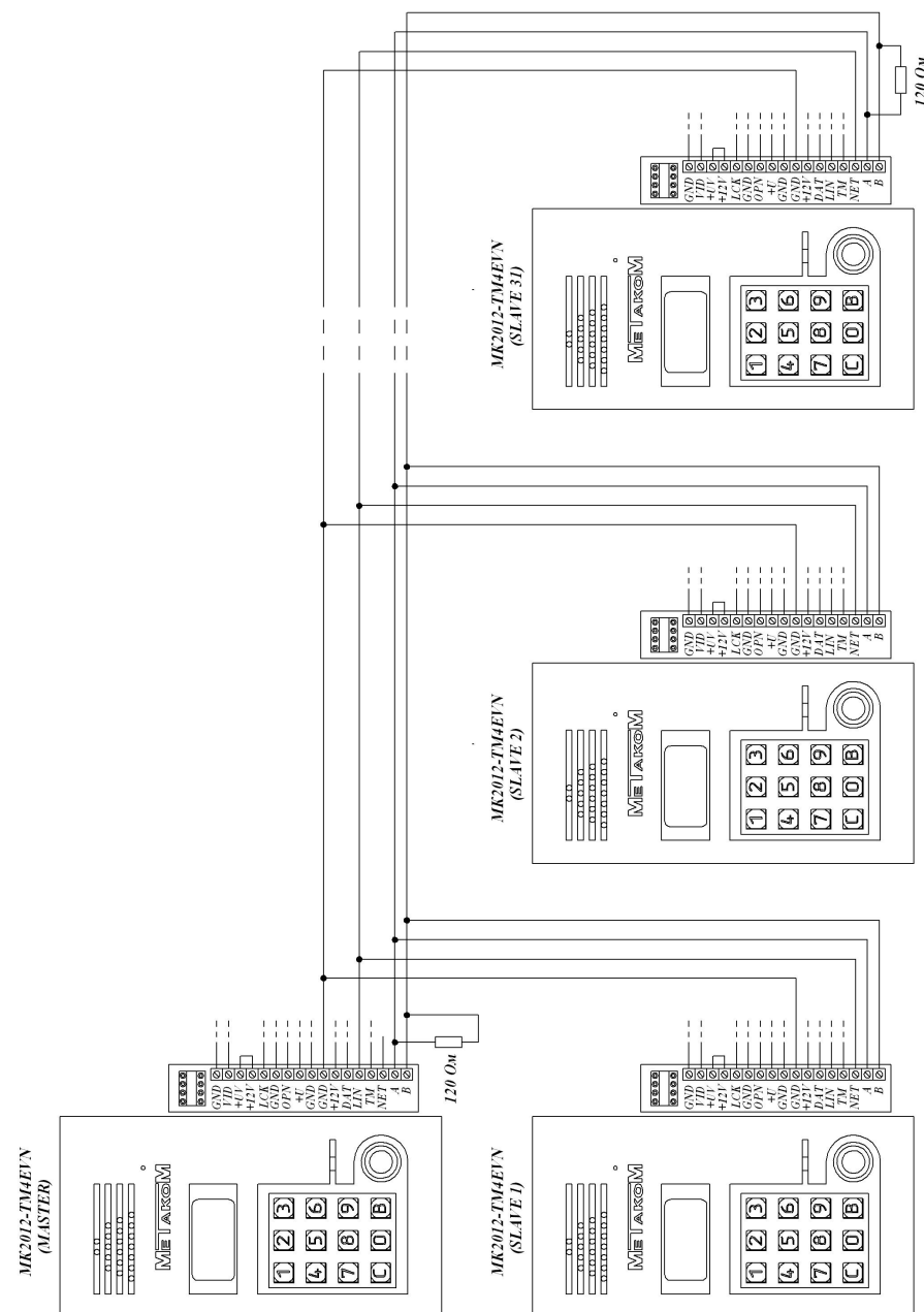
Рис. 3 Пример монтажа блока вызова МК2012-ТМ4ЕVN для огороженных территорий с одним входом на территорию.
